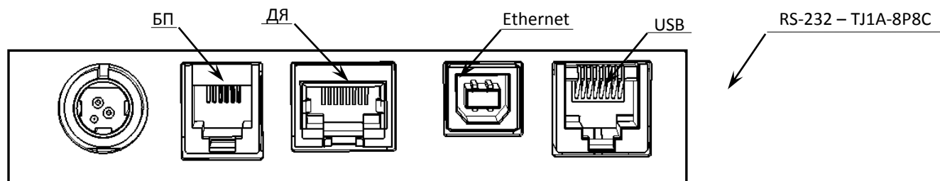
Рисунок 3. Разъемы для подключения внешних устройств к ККТ
