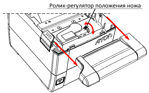
Рисунок 7. Ролик-регулятор положения ножа автоотрезчика
