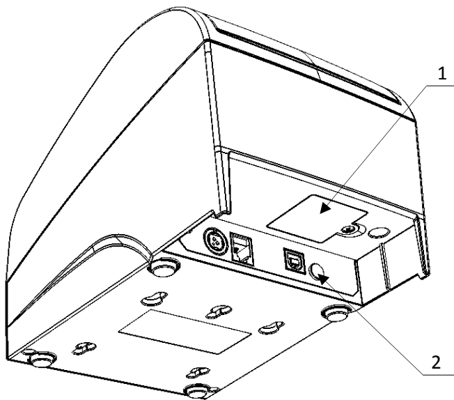
Рисунок 2. Вид сзади/снизу/справа
