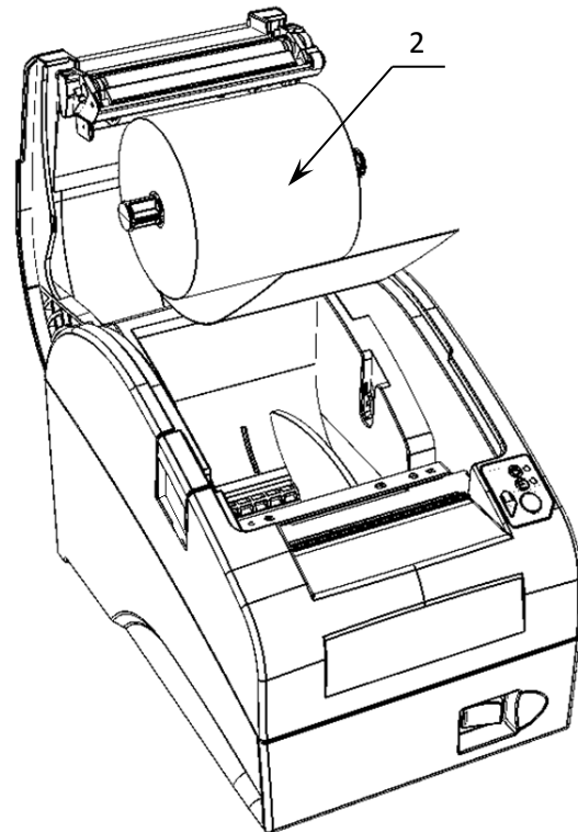
Рисунок 12. Установка ЧЛ
