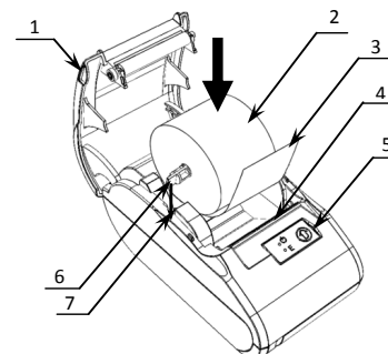
Рисунок 5. Заправка бумаги
