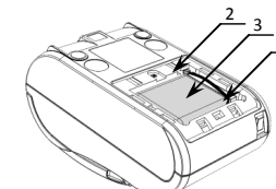
Рисунок 4. Подключение кабеля аккумуляторной сборки
